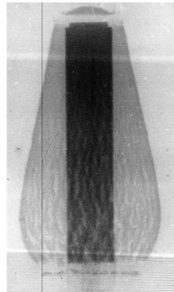
Рис. 2. Рентгенограмма процесса расширения оболочки и метания пластины при одностроннем инициировании
