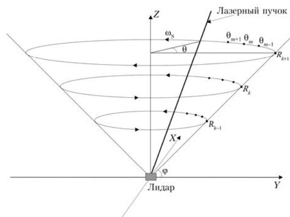
Рис. 1. Схема измерений импульсным КДЛ
