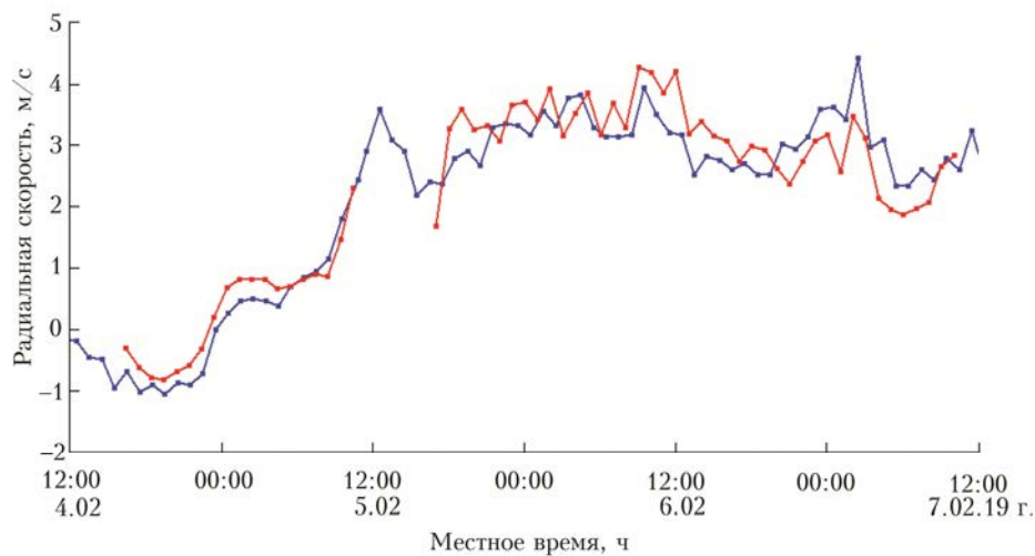
Рис. 4. Временные ходы радиальной скорости на расстоянии 442 м от лидара, полученные из измерений лидаром Stream Line (синяя кривая) и созданным в ИОА СО РАН макетом ветрового лидара (красная кривая)
