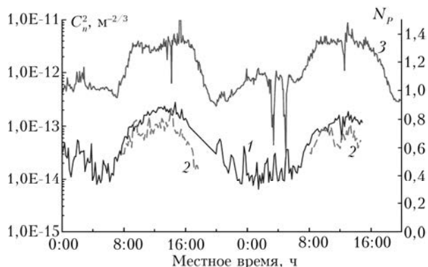
Рис. 6. Динамика изменения структурной постоянной флуктуаций показателя преломления, рассчитанная по данным акустических метеостанций (кривые 1 и 2), и временной ход коэффициента усиления обратного рассеяния на дистанции 500 м (кривая 3)
