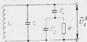
Рис. 2. Эквивалентная схема измерительной цепи.
