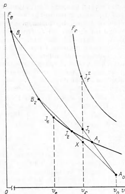
Рис. 1. Зависимость нормальных и пересжатых режимов детонации от \alpha . F_j, L_{\alpha_1}, L_{\alpha_2}, L_{\alpha_3} и J_j, J_1, J_2, J_e — соответствующие линии возврата и точки Жуге при \alpha = \infty, \alpha_1, \alpha_2, \alpha_3 ( \alpha_1 > \alpha_* > \alpha_2 > \alpha_{**} > \alpha_3 ).
