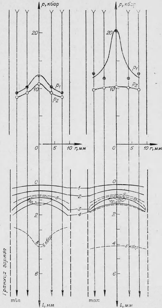
Рис. 3. Структура фронта идеальной детонации в заряде: с d=20 мм, p_1 — давление на вершине химика, p_2 — давление в плоскости Чепмена-Жуге.
