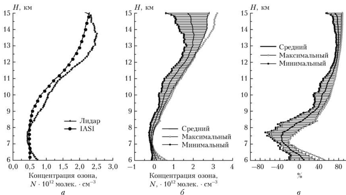
Рис. 3. Средние вертикальные профили озона и их различия: а – средние профили; б – различия концентраций, измеренных лидаром и IASI, в абсолютных единицах; в – относительные разности (лидар – IASI)/лидар
