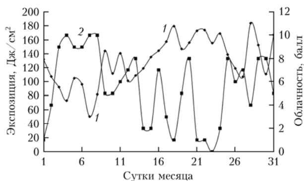
Рис. 2. Величины суточной энергетической экспозиции УФ-излучением Солнца (1) и облачности (2) в мае 2003 г.
