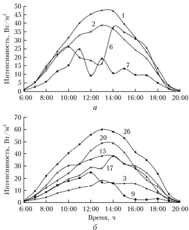
Рис. 1. Дневное изменение интенсивности УФ-излучения (290–400 нм): а – май 2003 г.; б – май 2004 г. (цифры у кривых соответствуют числу месяца)
